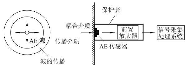
(c) 声发射监测原理示意图
