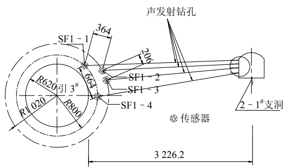
图 4 3-3 监测断面声发射传感器布置图(单位: mm) Fig.4 Location of AE sensors on section 3-3(unit: mm)
