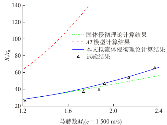
图 6 拟流体侵彻范围 ( 3.0 \geq M_a \geq 1.5 ) 内裂纹区半径计算结果与实验结果对比
