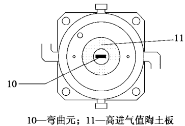
图 3 非饱和土底座结构示意图
