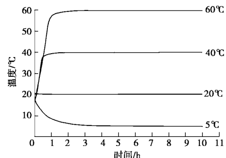
图 9 不同控温目标下内压力室温度与时间曲线
