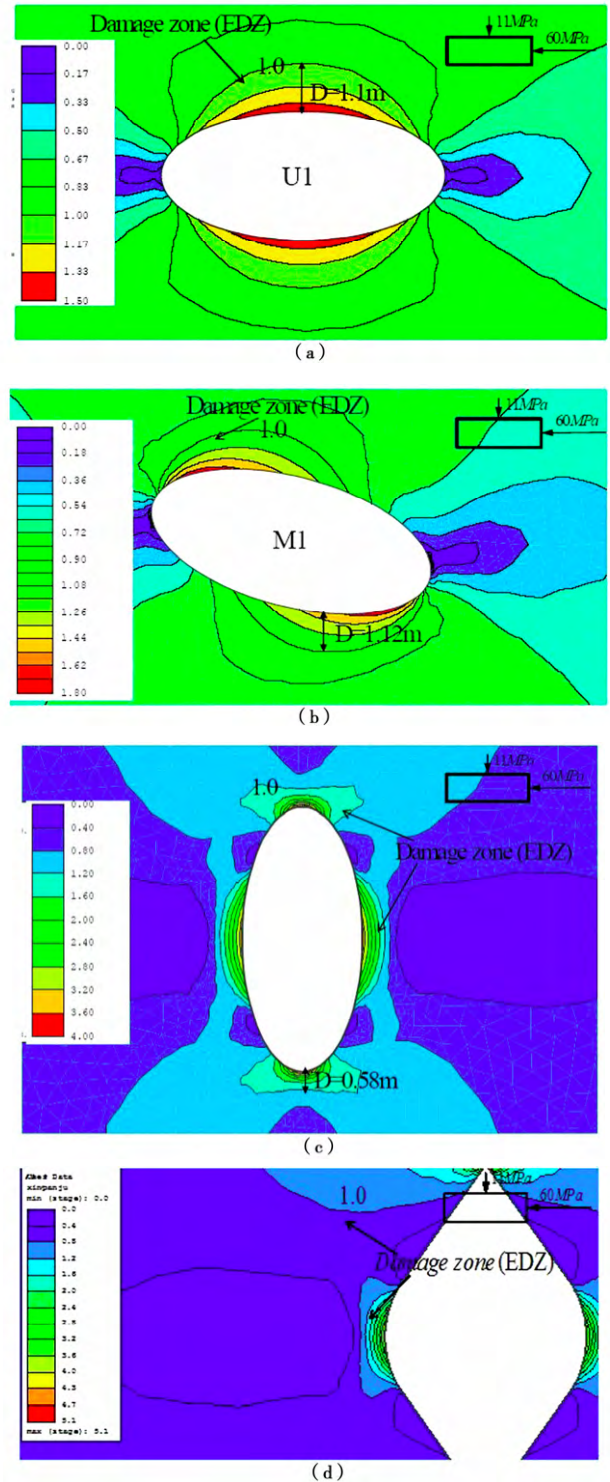
图 8 不同洞室断面损伤区云图对比
