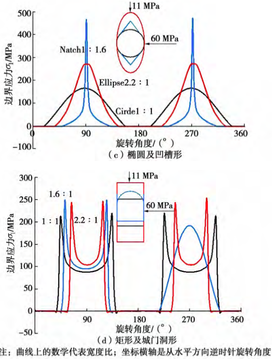
图 7 不同洞室断面边界切向应力对比
