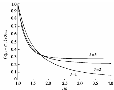
图 3 不同应力比下剪应力向围岩内部的衰减曲线
