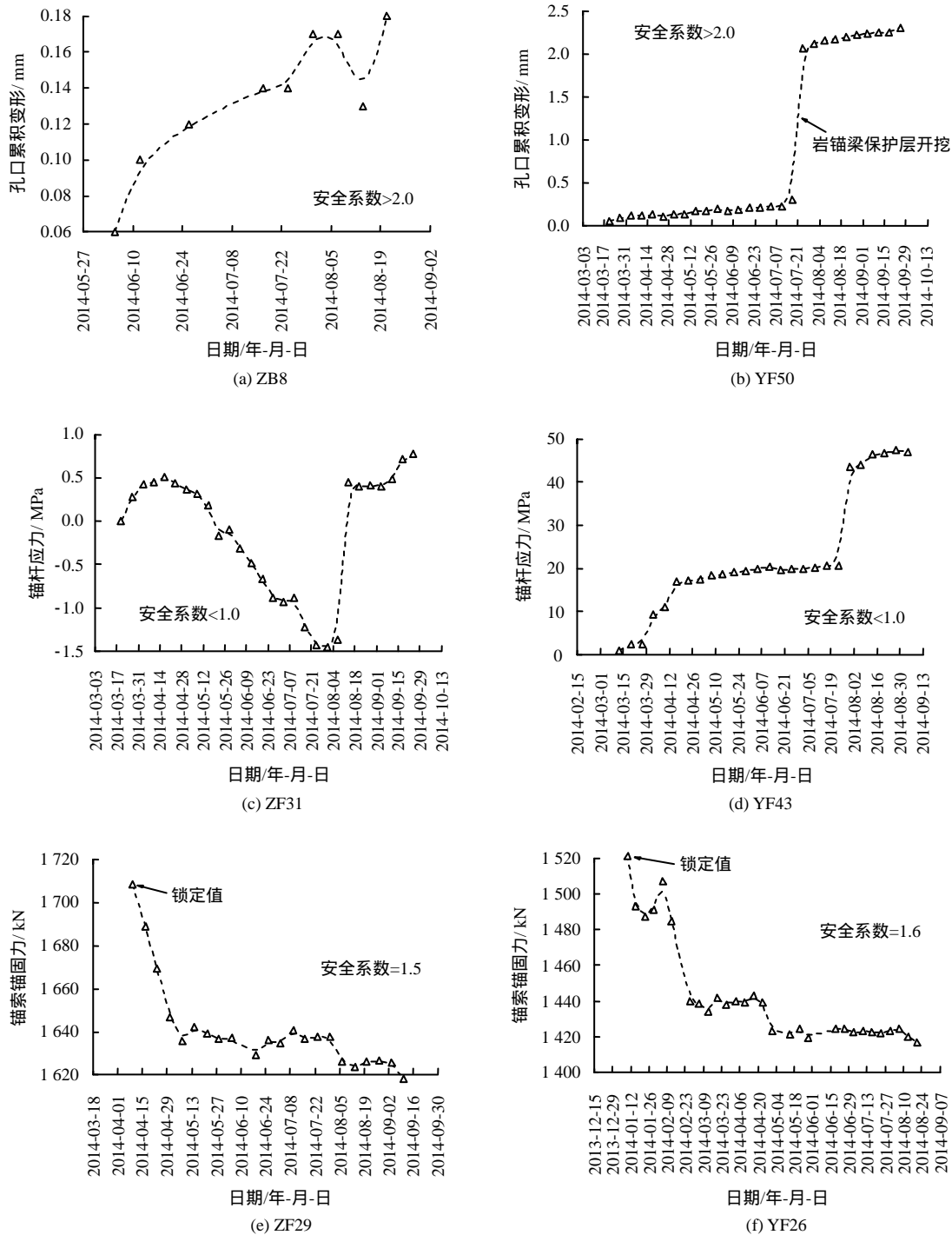
图6 块体监测时程曲线
