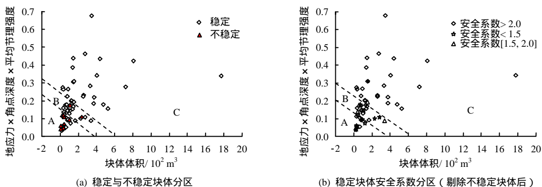
图 5 离散元强度折减法计算的安全系数统计
