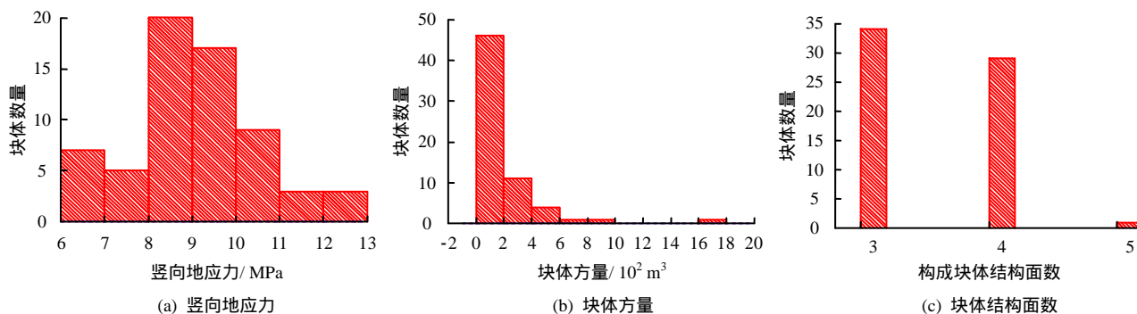
图 4 块体基本信息统计直方图
