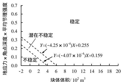
图 7 块体稳定性分区
