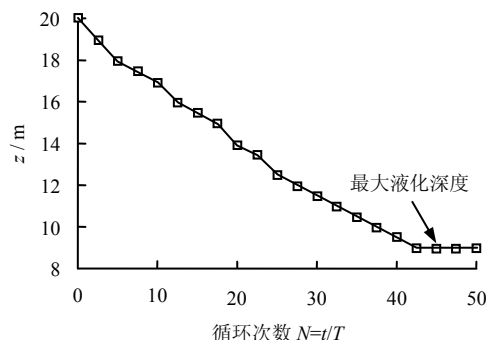
图 6 波浪作用下欠密实海床内液化区前缘深度的发展过程
