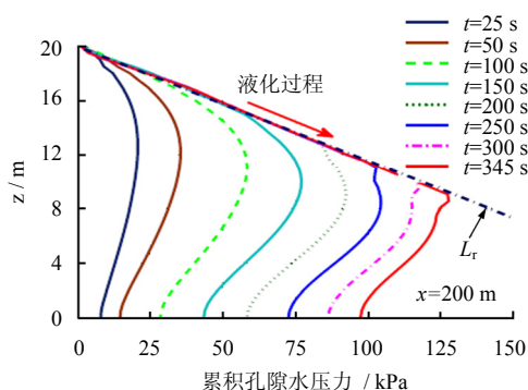
图 5 累积孔隙水压力沿海床深度在典型时刻的分布图
