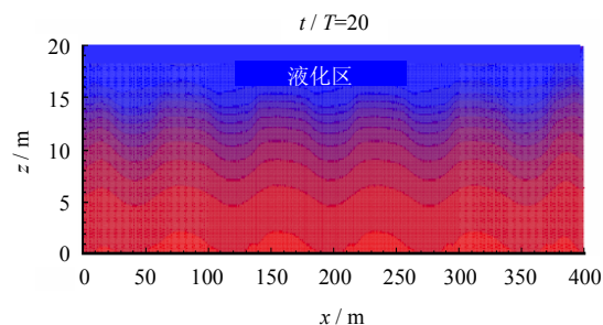
图 7 波浪作用 20 个周期后海床内的液化区范围
