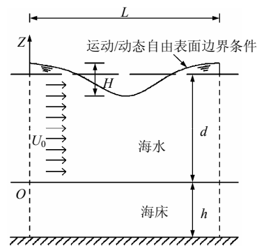
图 1 波浪作用下海床发生液化的计算概念图 Fig.1 Schematic of wave-induced liquefaction in loose sandy seabed
