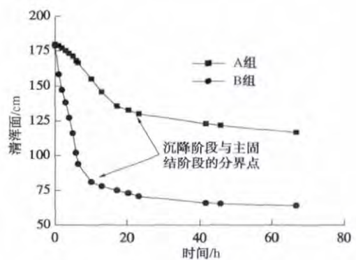
图6 清浑面随时间变化曲线（72 h）
