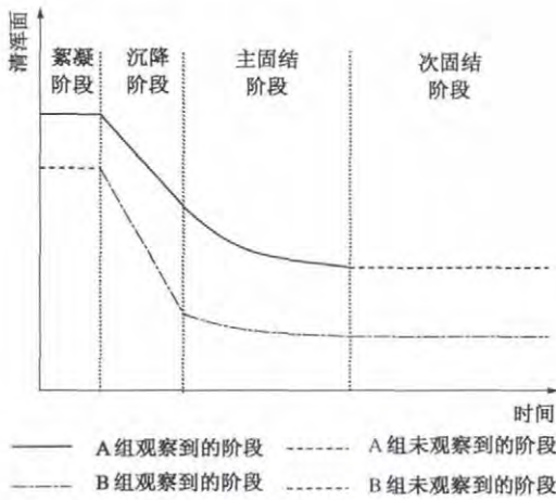
图 8 清浑面随时间变化曲线示意图
