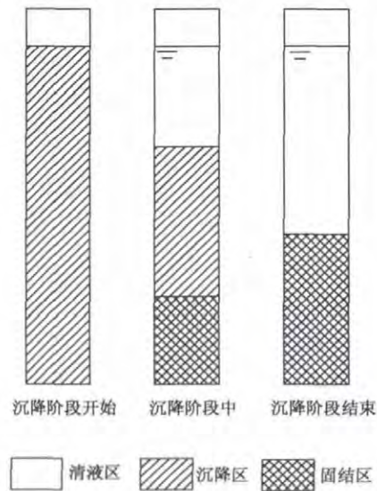
图 10 沉降阶段沉降柱内分区
