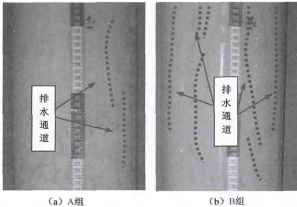
图 11 沉降过程中的树枝状通道
