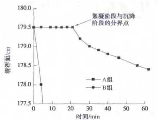
图5 清浑面随时间变化曲线（60 min）
