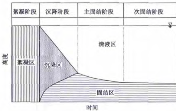
图 9 碱渣沉降示意图
