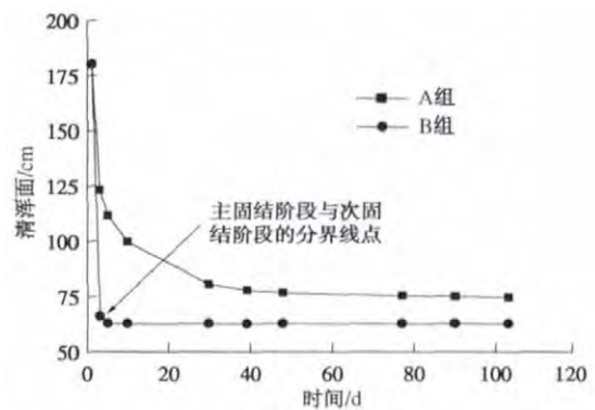
图7 清浑面随时间变化曲线（105 d）
