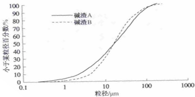
图 2 碱渣颗粒级配曲线
