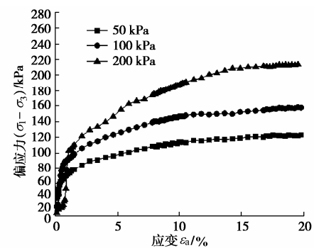
图 2 重塑软土三轴应力-应变关系
