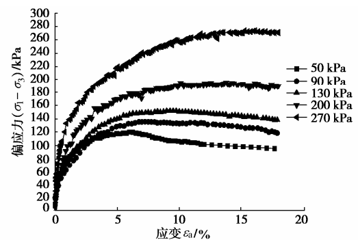
图 1 原状软土三轴应力-应变关系
