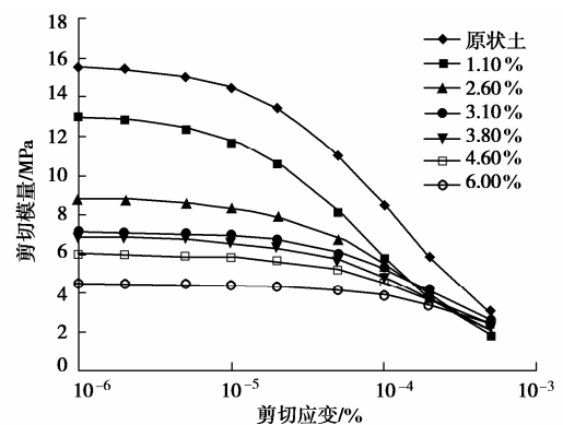
图6 共振柱试验获得的剪切模量与剪切应变关系
