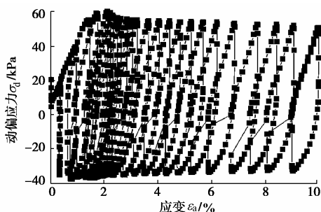
图4 动应力-应变曲线
