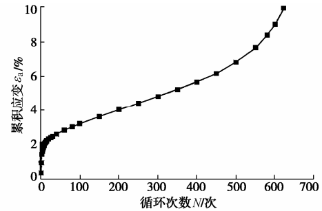
图5 轴向应变与循环次数的关系
