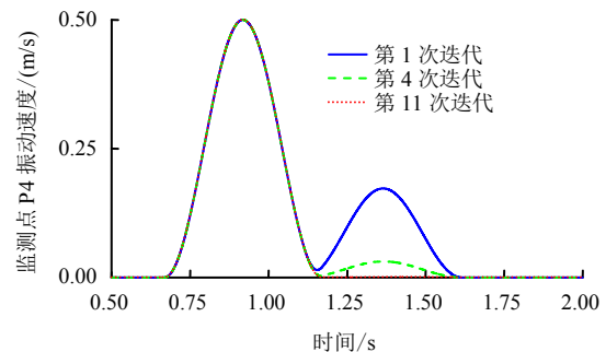
图 7 \beta_{2p} 取 0.5 初值条件下, 监测点 P4 振动速度时程 Fig.7 The velocity history of P4 when \beta_{2p} takes 0.5
