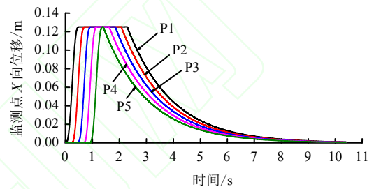
图 14 各监测点 X 向位移时程
