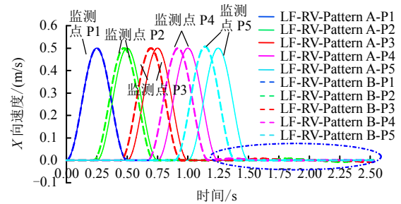
图 3 各监测点 X 方向速率
