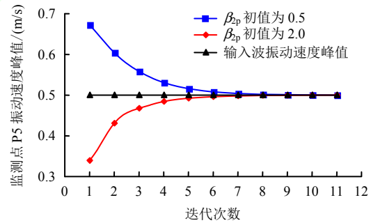
图 6 \beta_{2p} 取不同初值条件下, 右侧黏性边界监测点 P5 振动速度峰值随迭代次数变化 Fig.6 The velocity peak value of P5 on right viscous boundary varies with the number of iteration
