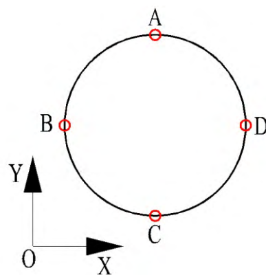
图5 假设的隧道设计轮廓线平面图 Fig.5 Assumptive tunnel design outline plan
