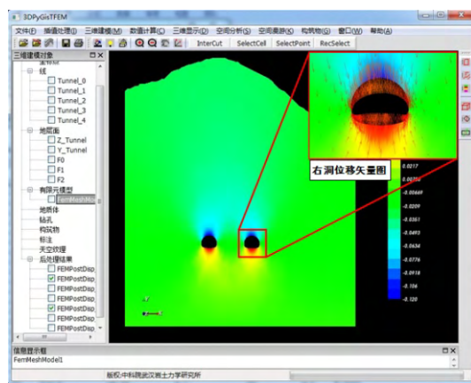
图 14 地质剖面 P1 位移计算结果图 Fig.14 Tunnel-induced displacement of geological section P1
