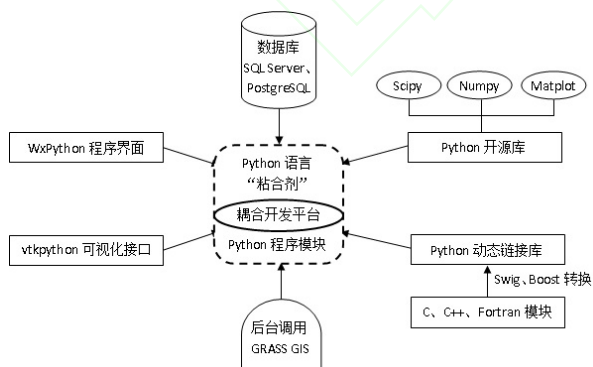
图 1 GRASS GIS 与有限元复合系统开发框架图
