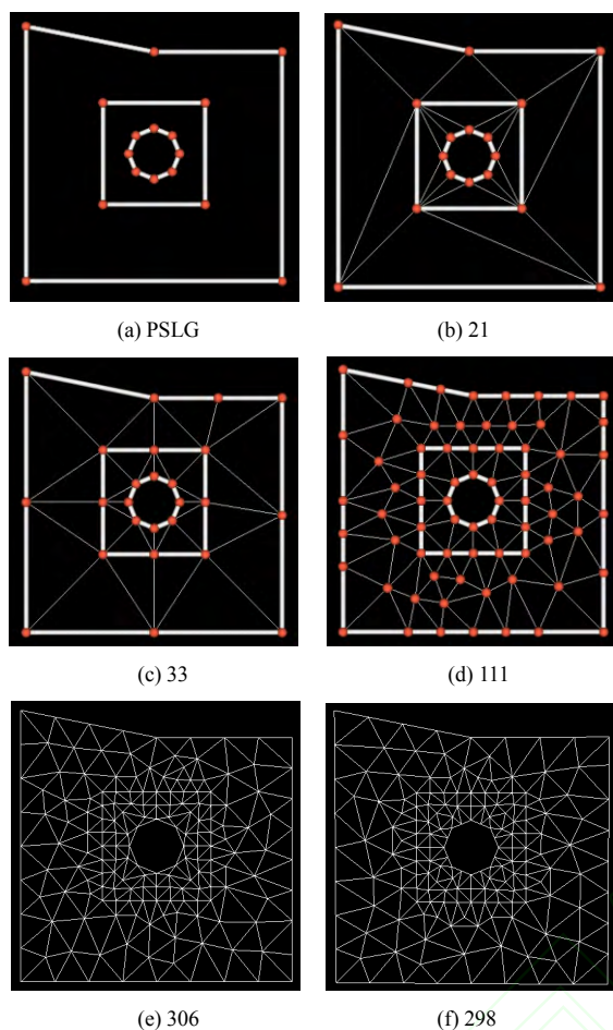
图9 不同约束条件下 Delaunay 剖分算法获得的三角形网格
