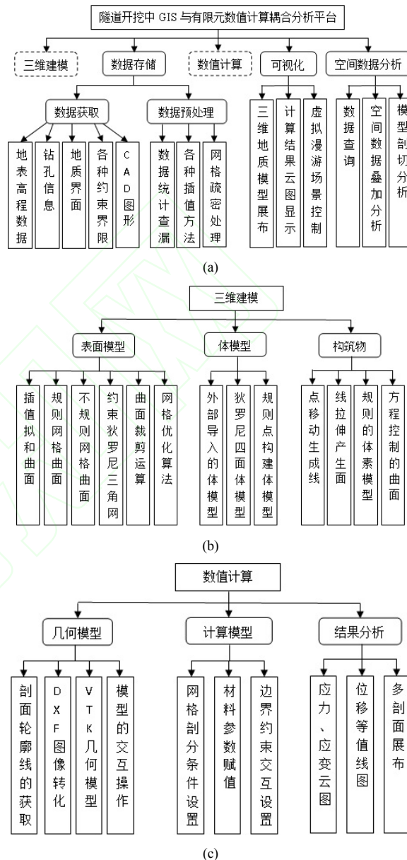
图 2 系统总体结构设计图
