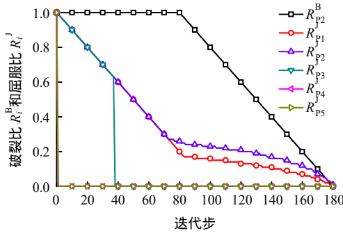
图 5 滑裂面的渐进破坏过程
