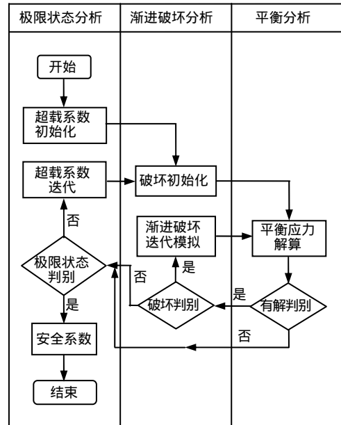
图 3 稳定性分析流程 Fig.3 Flow chart of stability analysis
