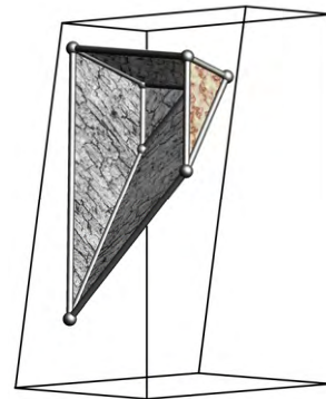
图 1 岩坡和块体的几何模型
