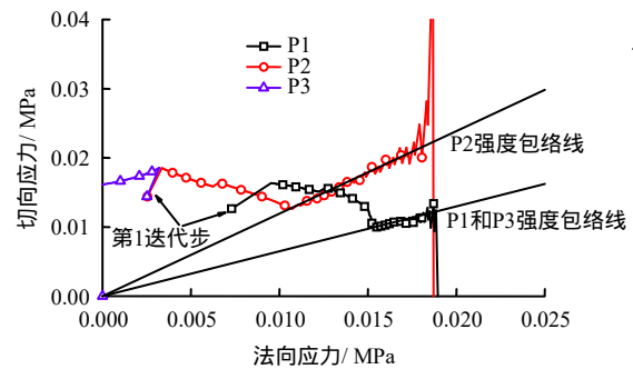
图 6 渐进破坏过程中裂隙面的的应力调整
