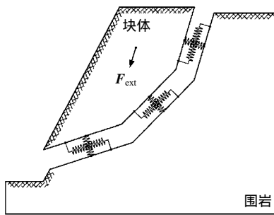
图 2 滑裂面的力系模型
